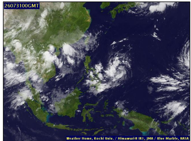
ภาพถ่ายดาวเทียม วันที่ ๓๑ ก.ค. ๒๕๖๙ เวลา ๐๗.๐๐ น.
