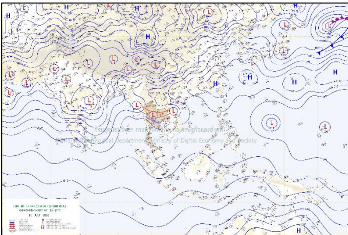
แผนที่อากาศ วันที่ ๓๑ ก.ค. ๒๕๖๙ เวลา ๐๑.๐๐ น.
